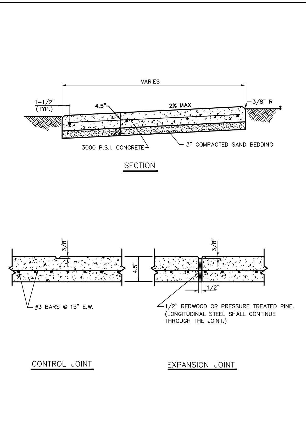
3 SIDEWALK DETAIL Scale: N.T.S. File:
