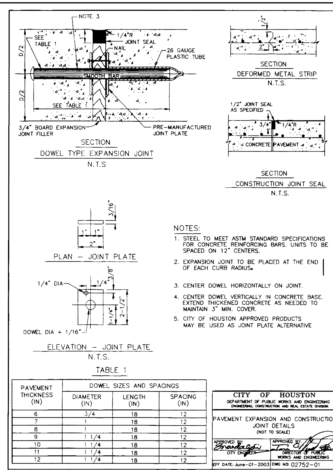
1 PVMT. JOINT DETAILS Scale: N.T.S. File:
