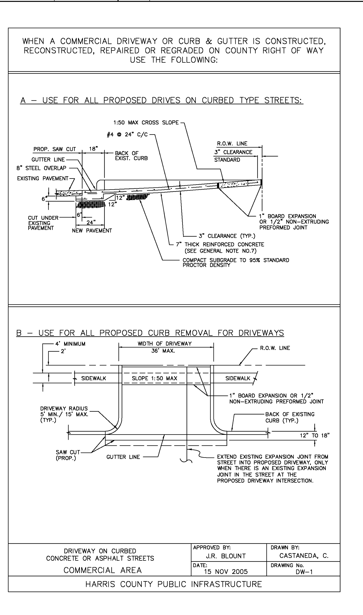
6 H.C. DRIVEWAY DETAIL Scale: N.T.S. File:
