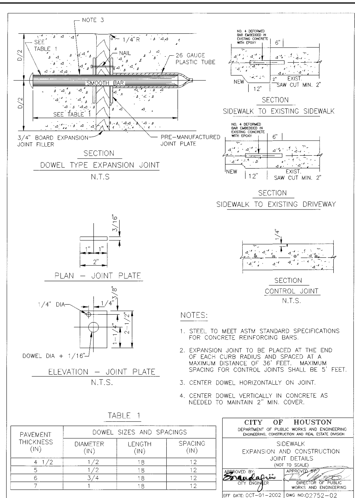
2 SIDEWALK JOINT DETAILS Scale: N.T.S. File:
