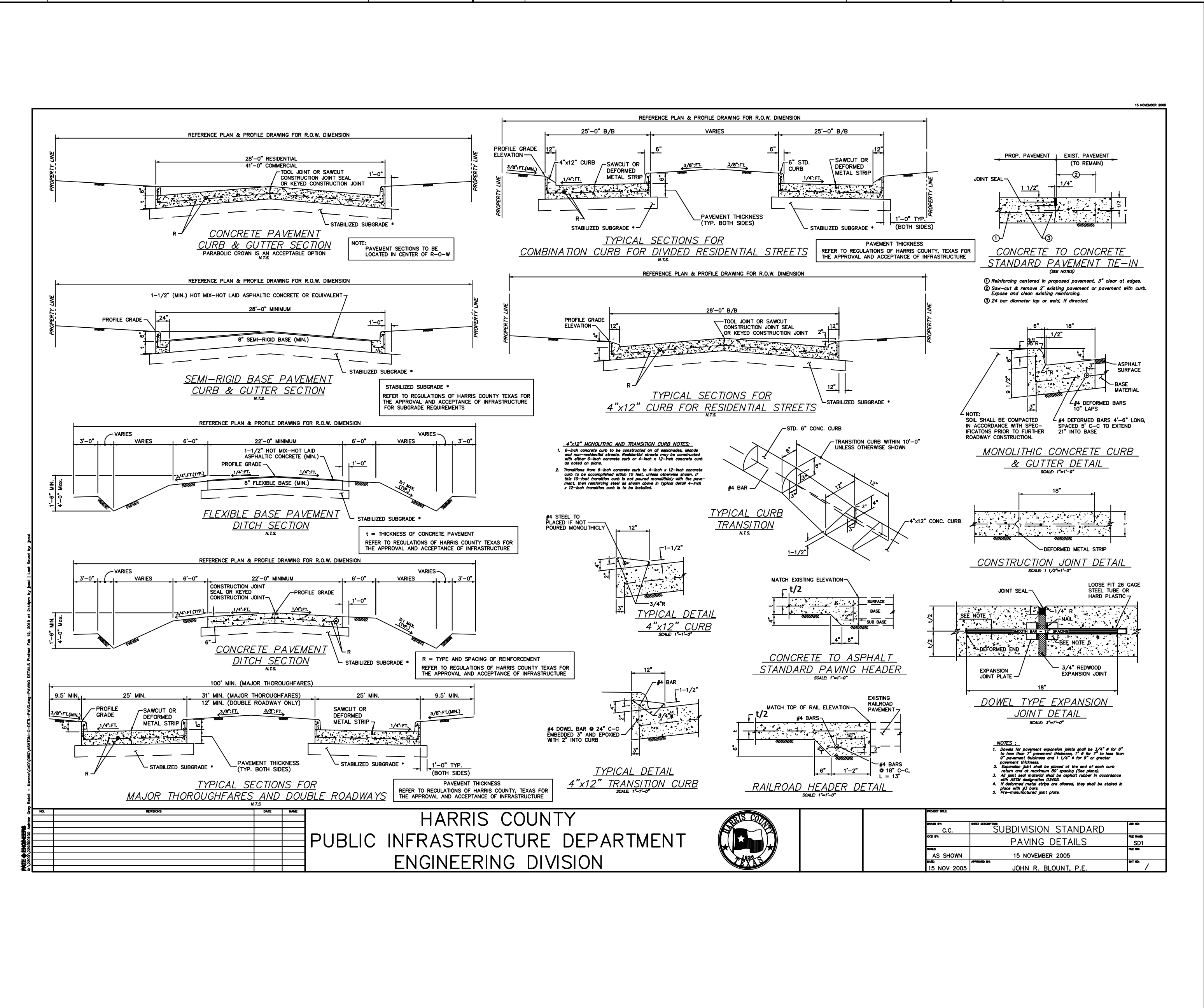
5 CURB/HEADER DETAIL Scale: N.T.S. File:
