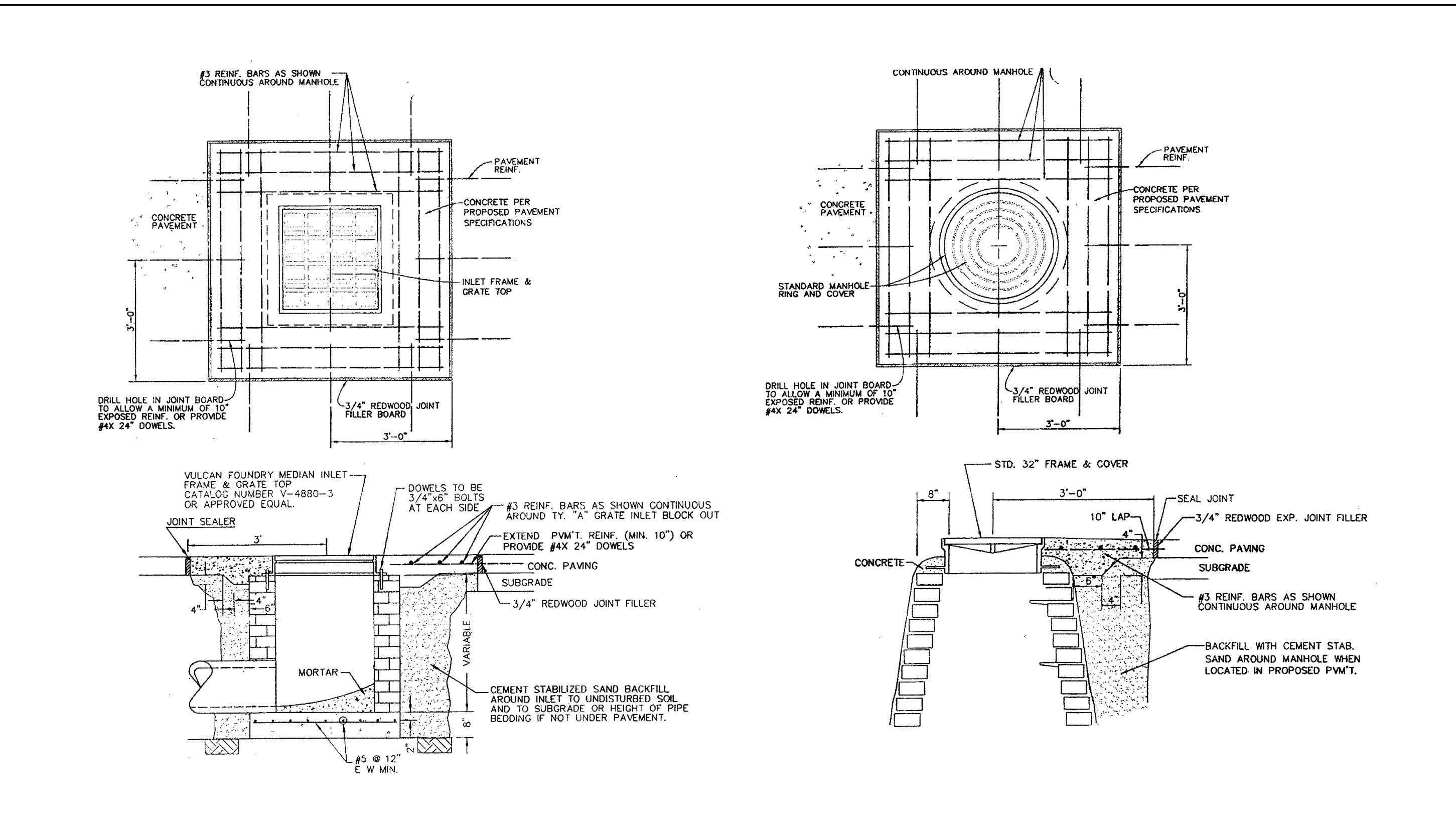
4 MANHOLE AND INLET BLOCKOUT Scale: N.T.S. File:
